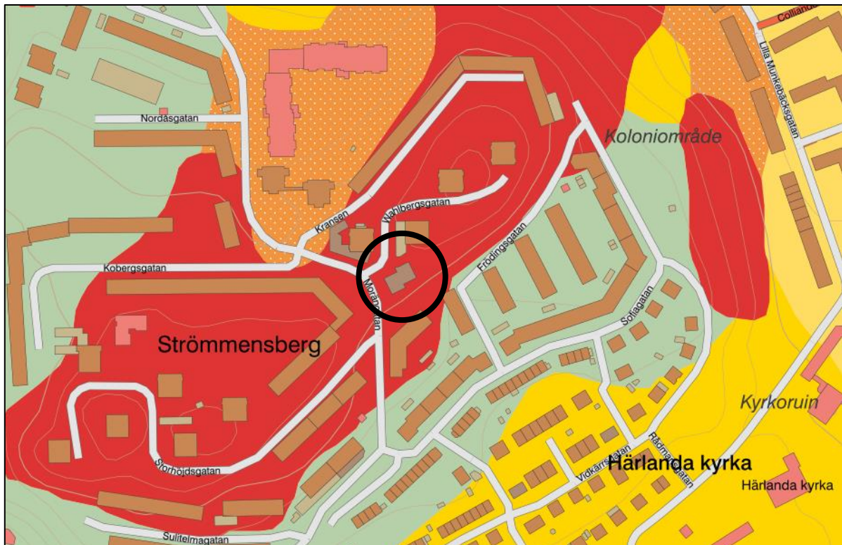
Figur 3. SGU:s jordartskarta. Svart cirkel visar läge för aktuellt undersökningsområde. Rött område visar läge för berg i dagen. Orange-markerat område visar läge för sand. Grönt område visar läge för morän omväxlat med sorterade material. Gult område visar läge för lera (Källa: SGU 2022).
